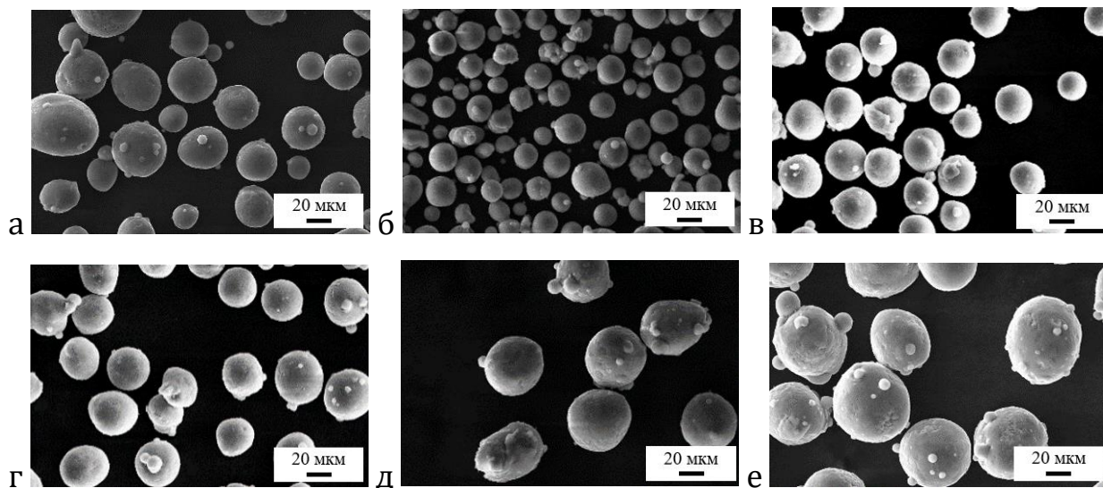
Рисунок 1 – Микроснимки стандартного порошка AlSi10Mg (а) и его просеянных фракций П1 (б), П2 (в), П3 (г), П4 (д), П5 (е)
