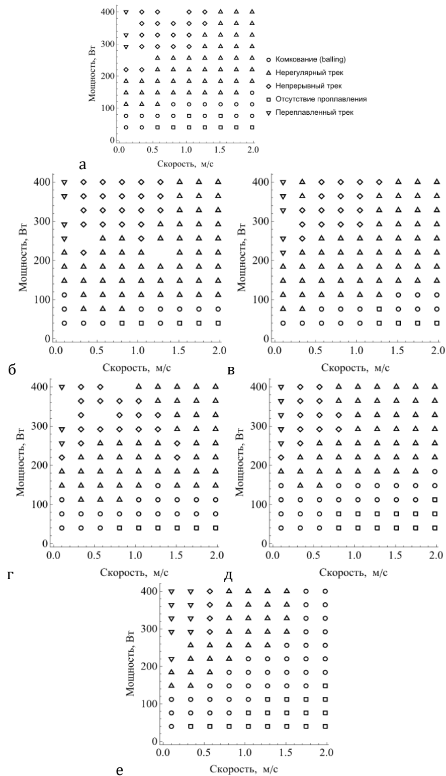
Рисунок 3 – Карты процесса, построенные по результатам анализа вида сверху: П0 (а), П1 (б), П2 (в), П3 (г), П4 (д), П5 (е)
