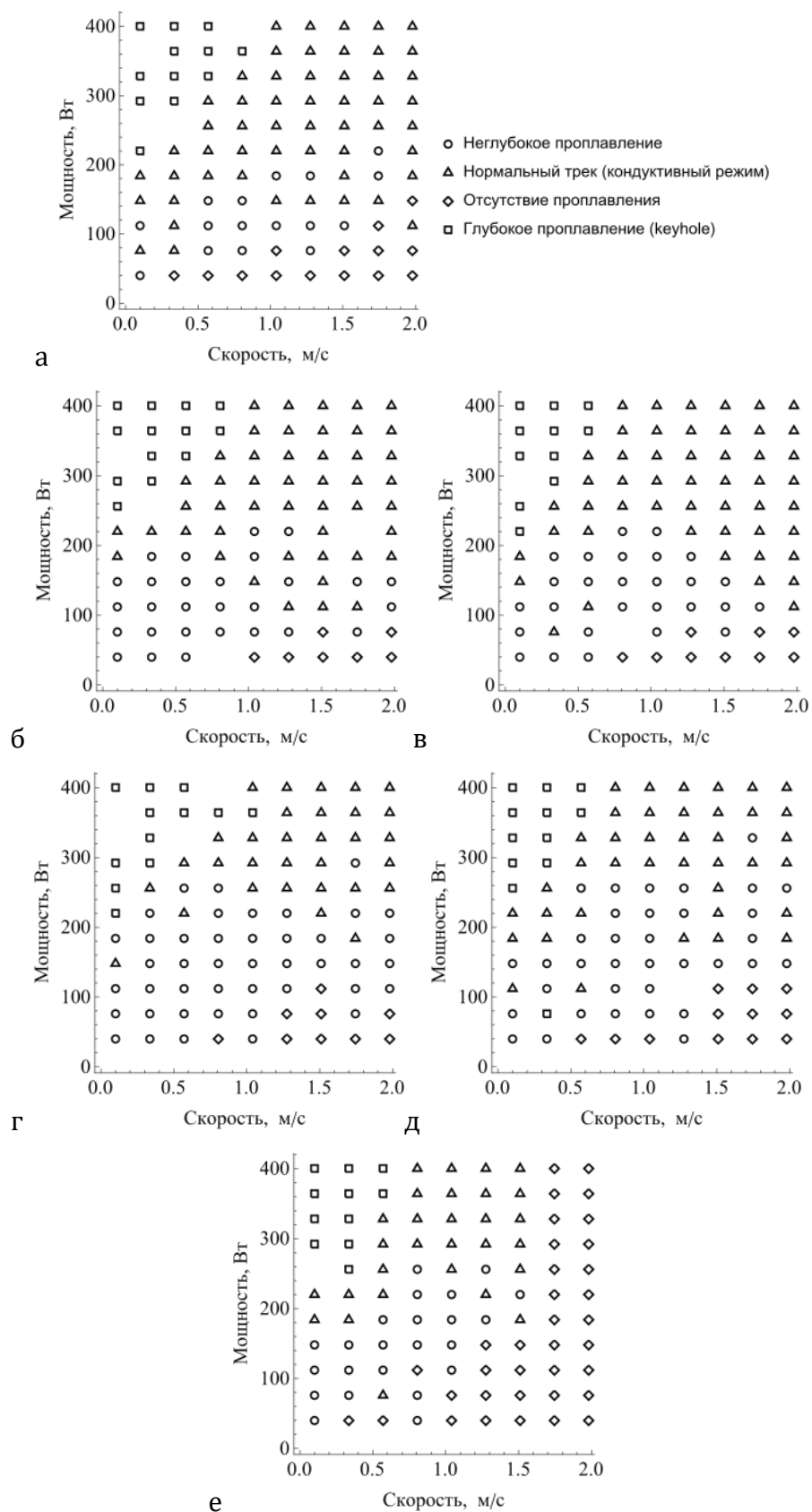
Рисунок 4 – Карты процесса, построенные по результатам анализа поперечных шлифов: П0 (а), П1 (б), П2 (в), П3 (г), П4 (д), П5 (е)
